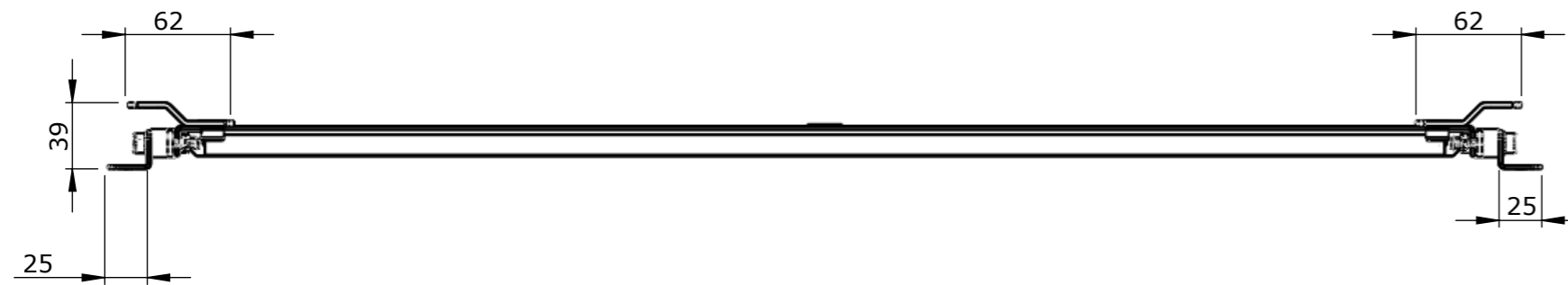
SECTION A-A SCALE 1 : 4
